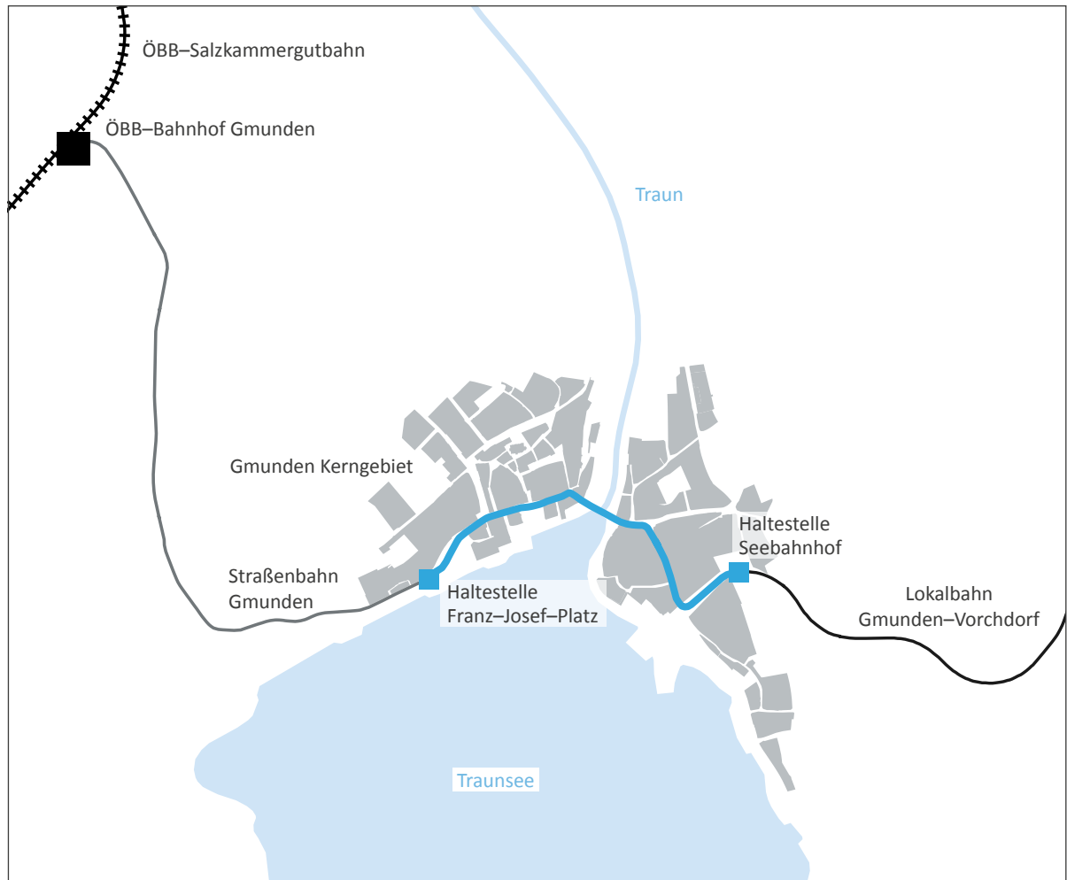
Abbildung 2: Durchbindungsprojekt Traunseetram
